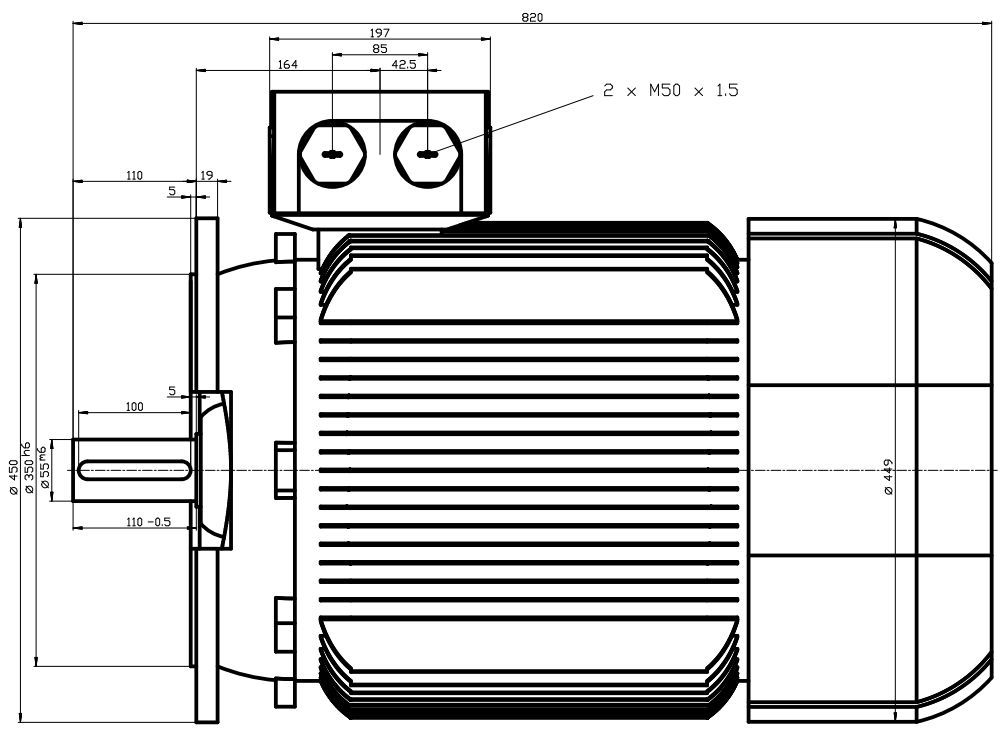
DIN332-DS M20 DIN 6085 Teil1
